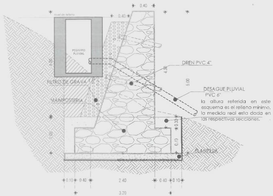
DETALLE DE MURO 3 S/ESC
