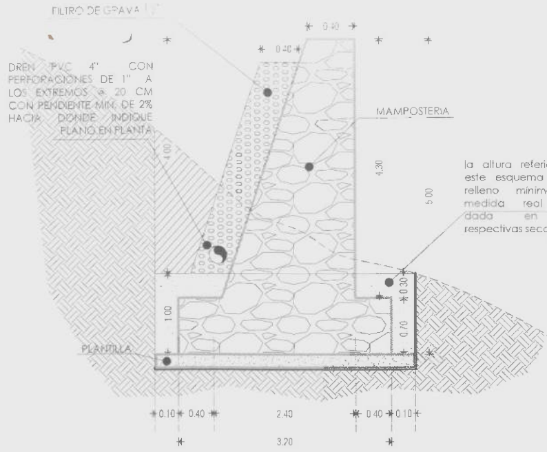
DETALLE DE MURO 2 S/ESC
