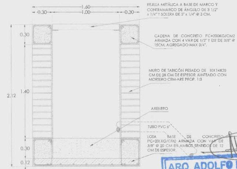
DETALLE DE REJILLA S/ESC
