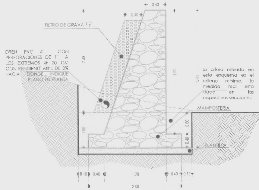
DETALLE DE MURO 4 S/ESC
