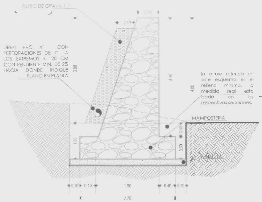
Detalle de muro con dren de pvc longitudinalmente al muro
