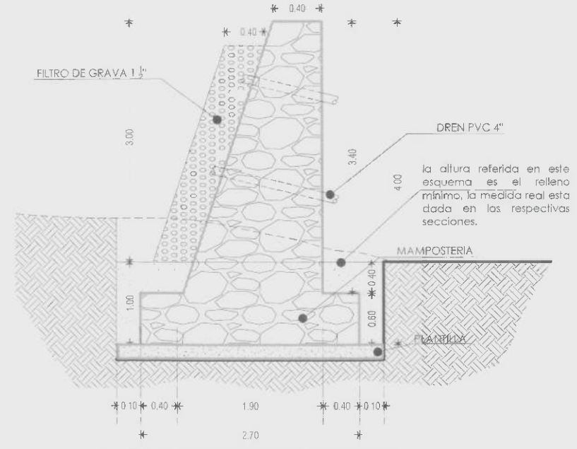
Detalle de muro con dren perpendicular al muro
