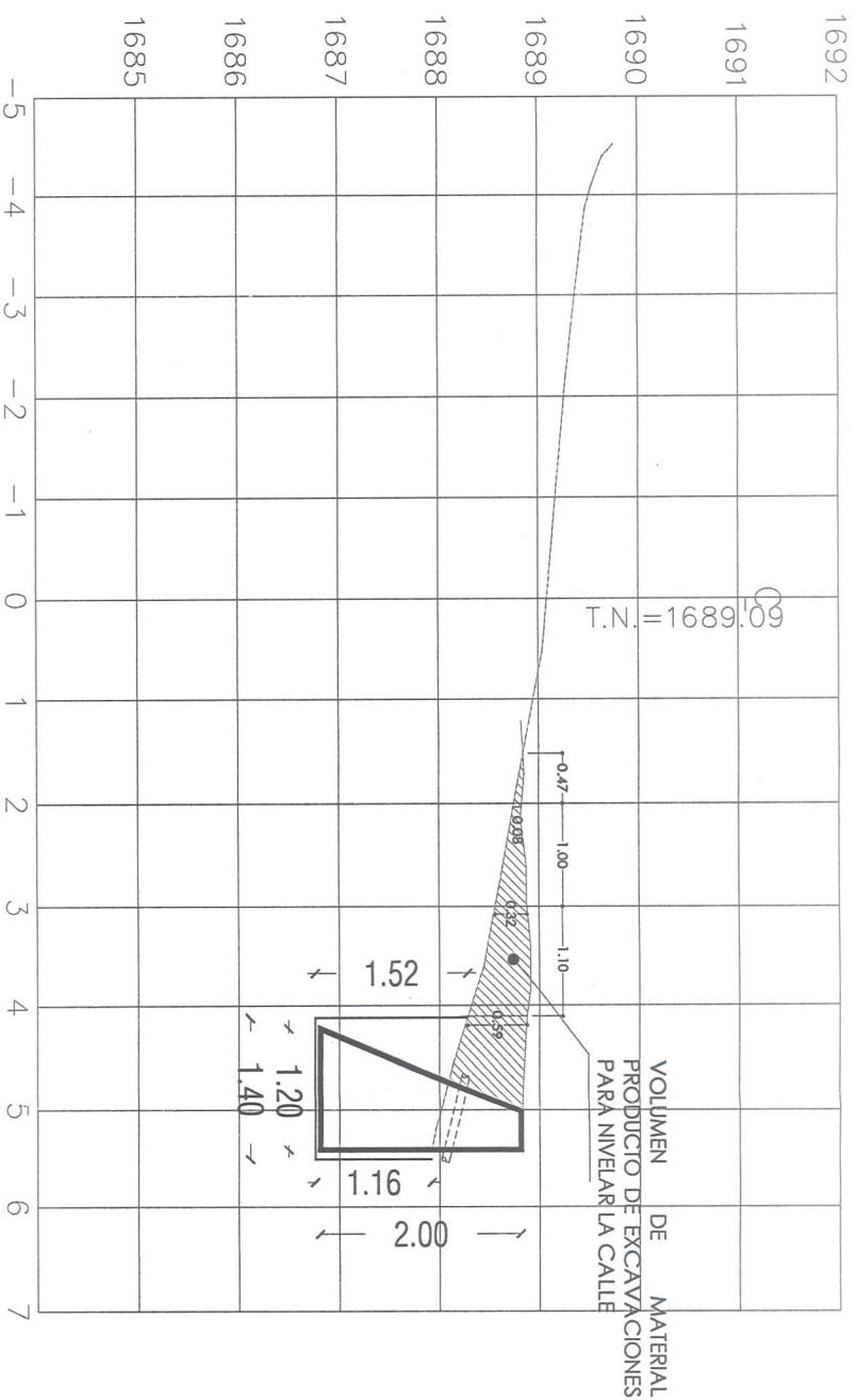
ESTACION 0+073.65 ESCALA HORIZONTAL 1 : 100 ESCALA VERTICAL 1 : 100
