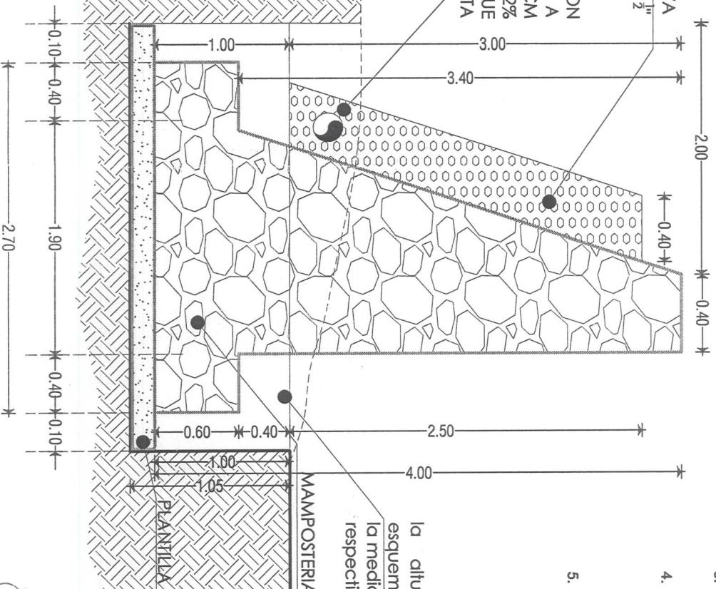
SECCIÓN DE MURO 4 S/ESC
