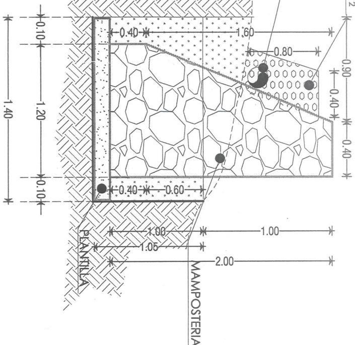
SECCIÓN DE MURO 2 S/ESC
