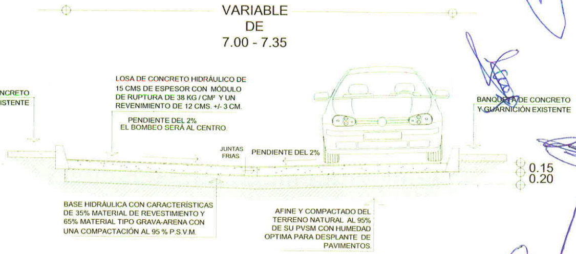
SECCIÓN DE CALLE CORTE A-A' 0+000.00 - 0+328.01
