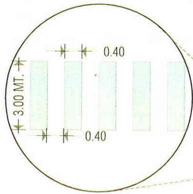
DETALLE DE LINEAS DE TRAFICO (MARIMBA)
