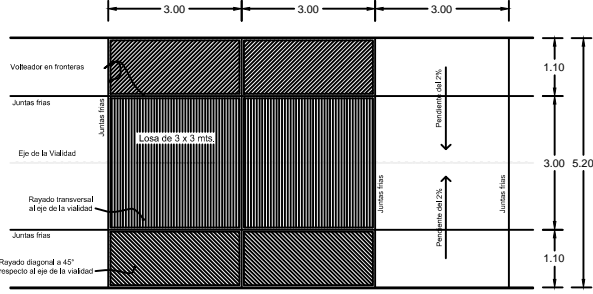
ESQUEMA DE DISTRIBUCIÓN DE LAS LOSAS DE PAVIMENTO (PLANTA) S/ESC.
