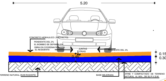
SECCIÓN TRANSVERSAL DE VIALIDAD B-B' s/esc
